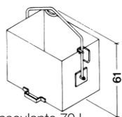
benne basculante 70 l
