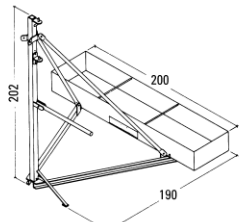
trepid pour montage sur toit plat avec caisse à lest 1863
