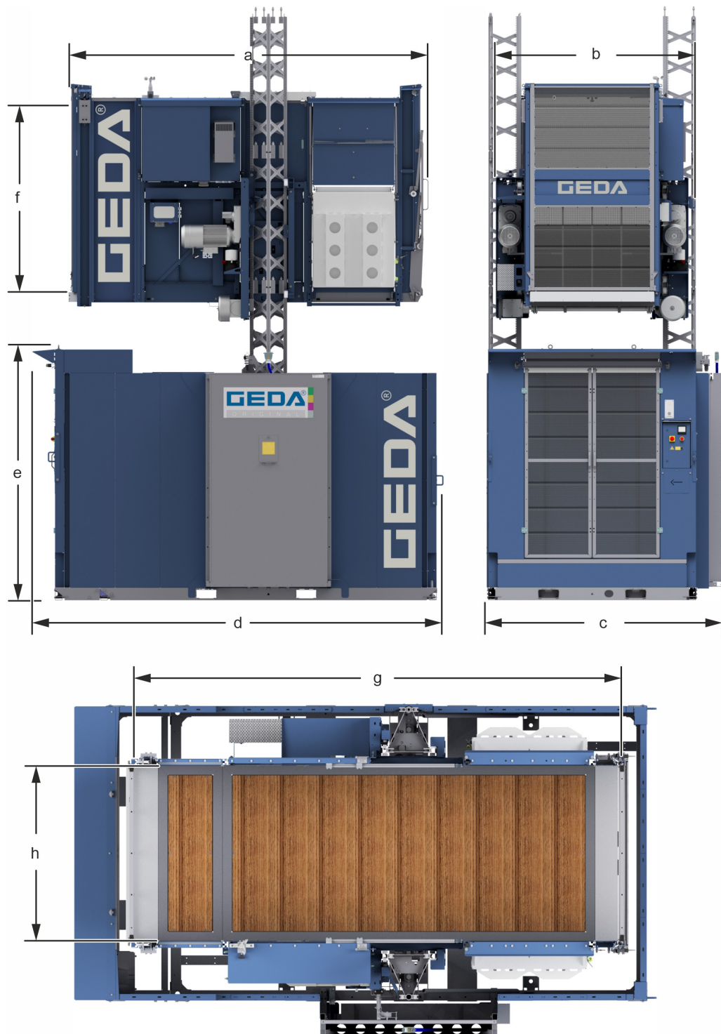
Abb. 5: Maße für Bühne E
