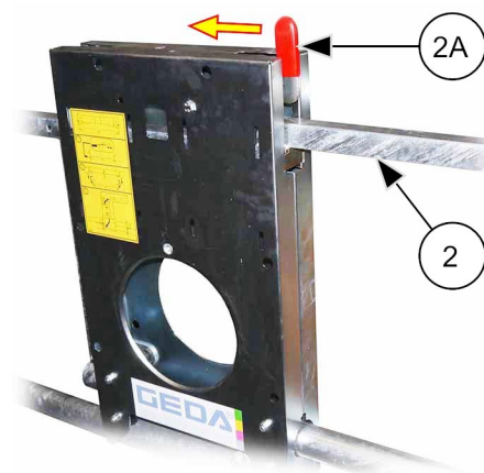
Abb. 25: Etagensicherungstür "Comfort" öffnen/schließen
