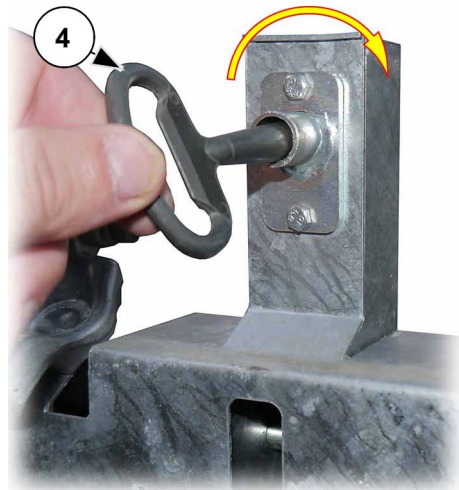
Abb. 28: Notentriegelung der Etagensicherungstür
