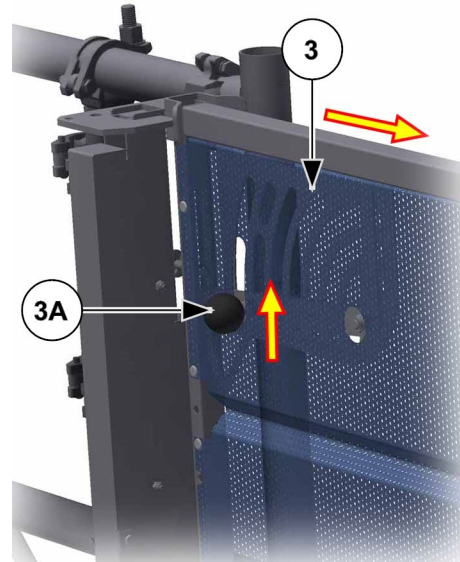
Abb. 27: Etagensicherungstür "VARIO" öffnen/schließen
