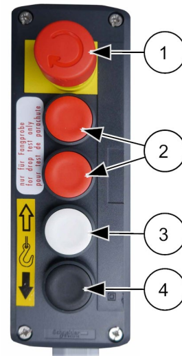
Abb. 40 Fangprobensteuerung
