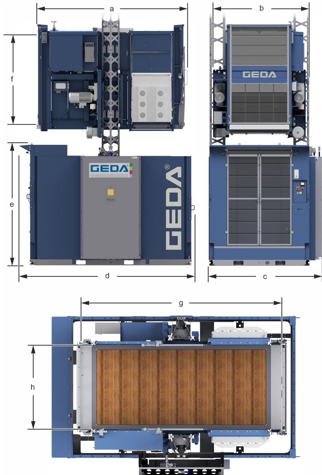
Abb. 4: Maße für Bühne D
