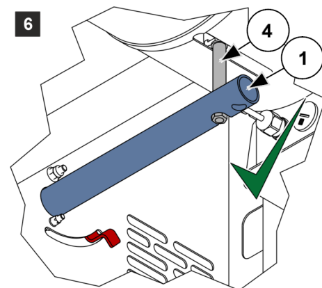
Abb. 70: Hebel am Bremslüfthebel ansetzen
