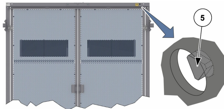
Abb. 32: Notentriegelung der Etagenflügeltür
