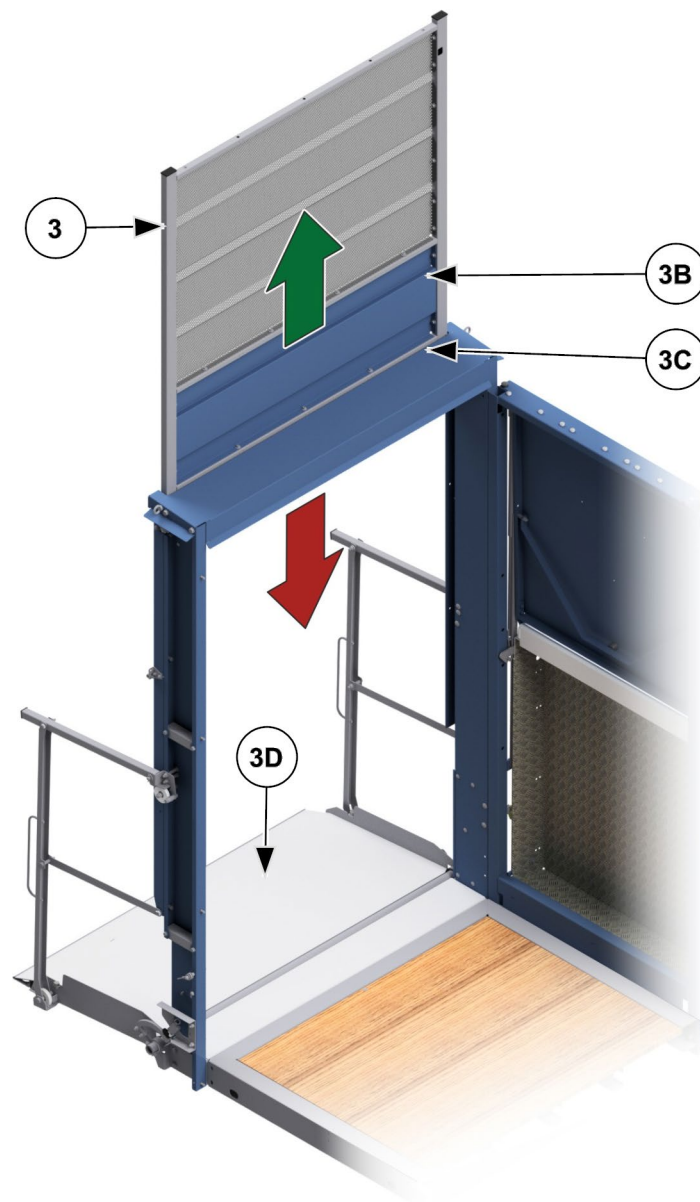
Abb. 15: Vertikale Schiebetür von innen
