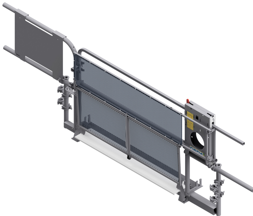
Abb. 24: Etagensicherungstür "Comfort" geschlossen (Füllblech)
