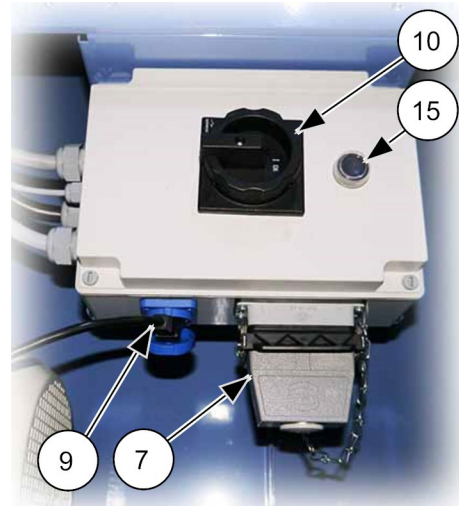
Abb. 39: Steuerung für Sonderbetrieb einstecken
