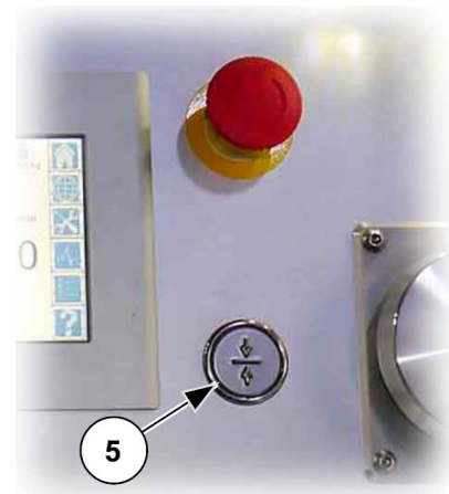
Abb. 64: Rückholbetrieb Fahrkorbsteuerung
