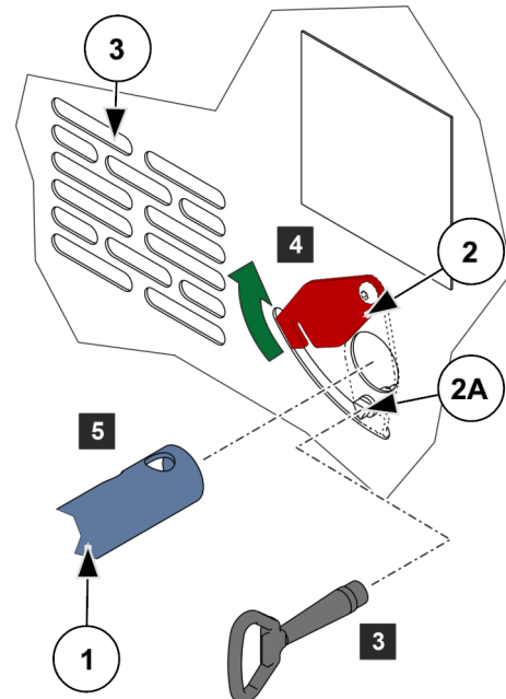
Abb. 69: Hebel zur Motorbremse führen
