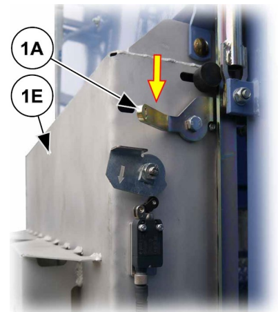
Abb. 75: Montagegesteg außen öffnen
