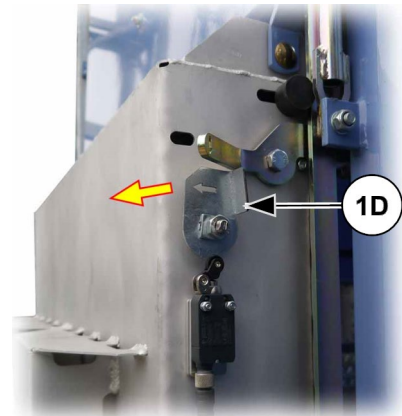
Abb. 74: Montagegesteg außen entriegeln
