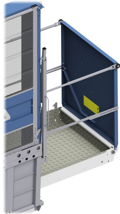
Abb. 73: Montagesteg geöffnet
