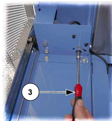
Abb. 16: Notentriegelung im Fahrkorb
