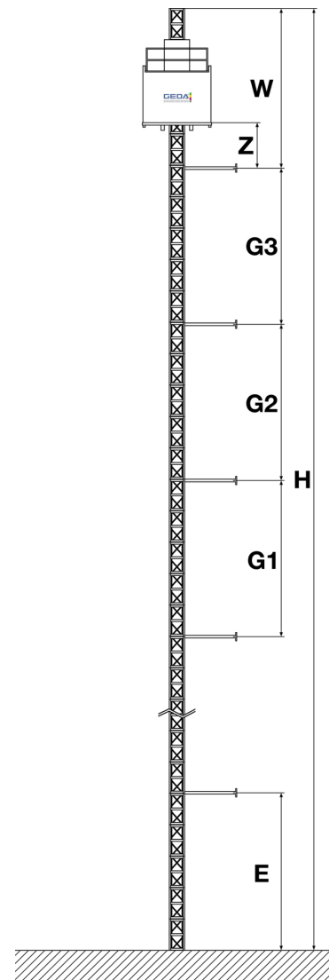
Abb. 3: Verankerung schematisch
