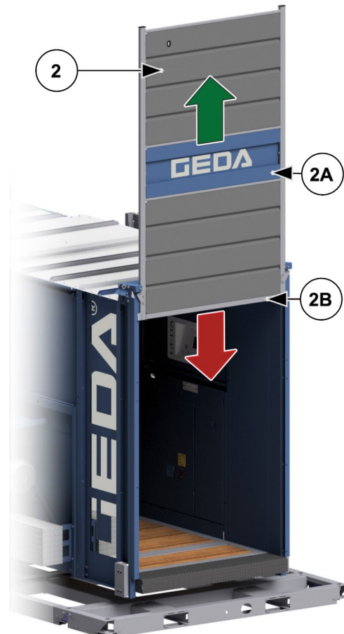
Abb. 13: Vertikale Schiebetür
