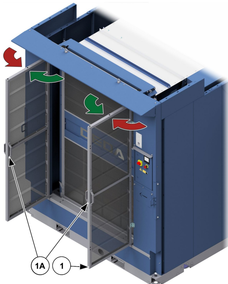
Abb. 11: Flügeltüren der Bodenumwehrung
