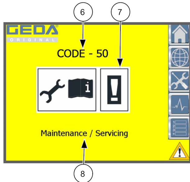
Abb. 58: Touch Display Wartung
