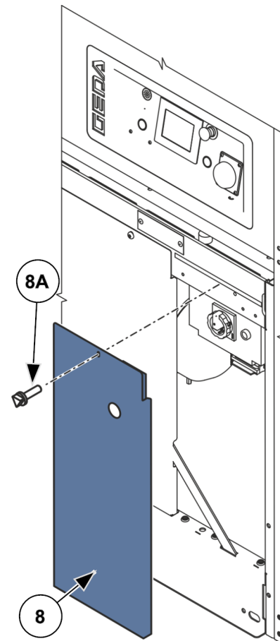
Abb. 38: Verkleidungsblech demontieren
