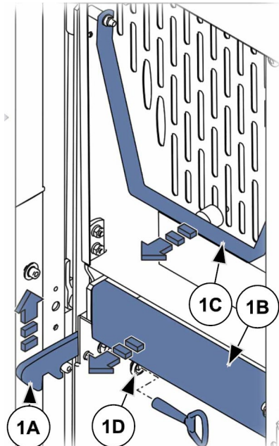
Abb. 72: Montagegesteg von innen öffnen
