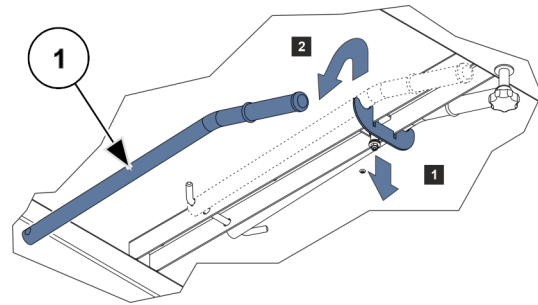
Abb. 68: Halterung für Hebel zum Bremsenlüften
