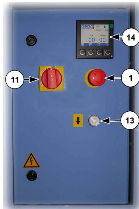
Abb. 33: Bodensteuerung
