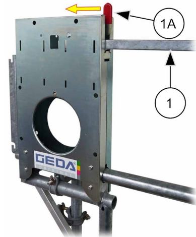
Abb. 21: Etagensicherungstür "Standard" öffnen/schließen
