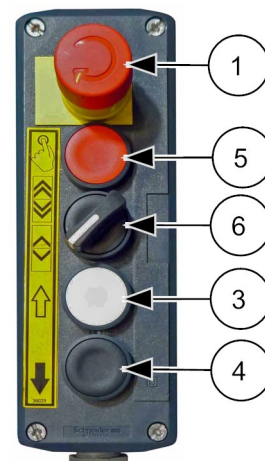
Abb. 41 Montagesteuerung
