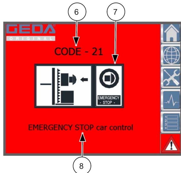
Abb. 59: Touch Display Störung
