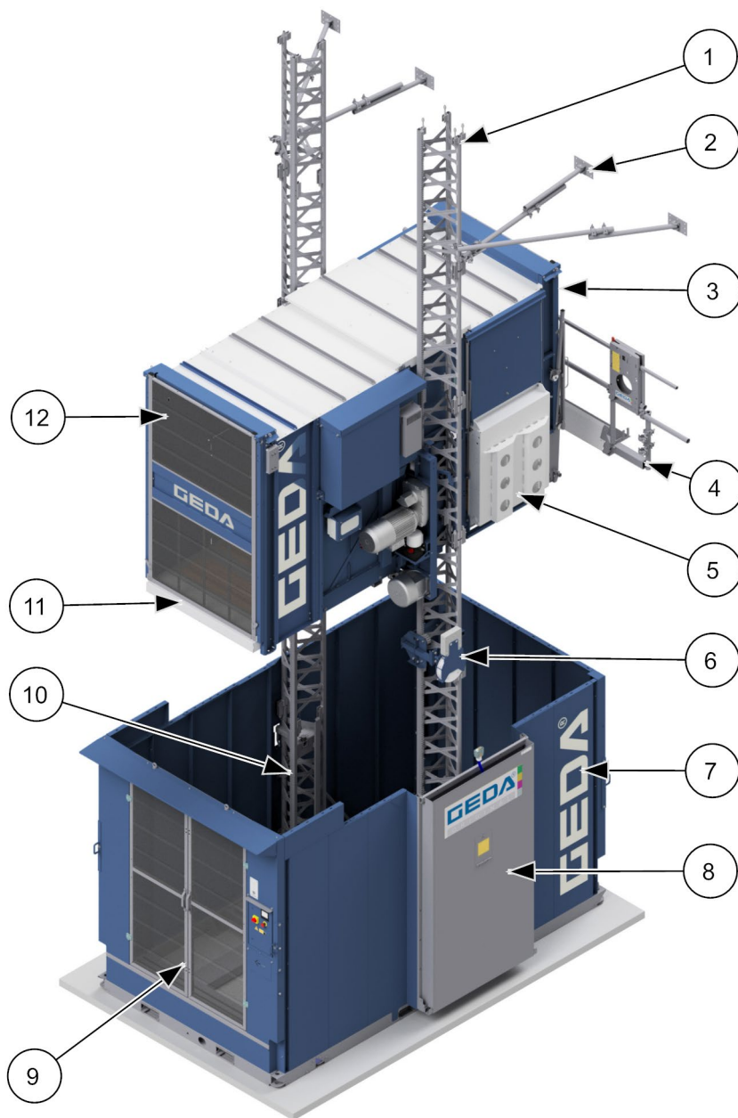
Abb. 9: Multilift P18 Übersicht
