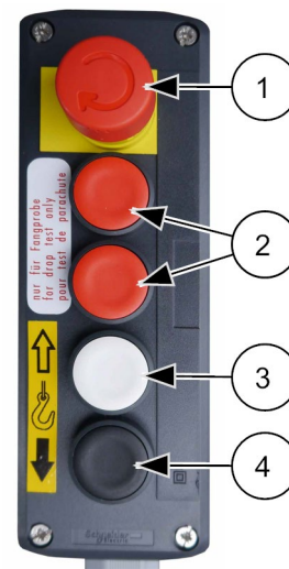
Abb. 62 Fangprobensteuerung zum Freifahren
