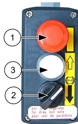
Abb. 60: Fangprobensteuerung
