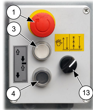
Abb. 55: Bodensteuerung für Umwehung (AUTOMATIK)
