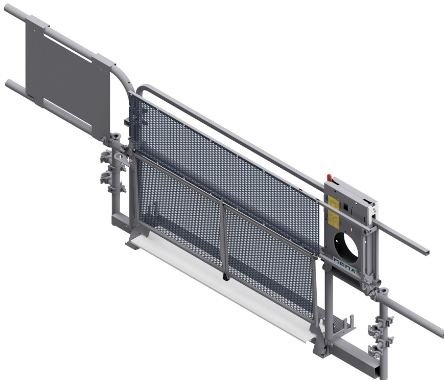
Abb. 45: Etagensicherungstür "Comfort" geschlossen (Füllblech)
