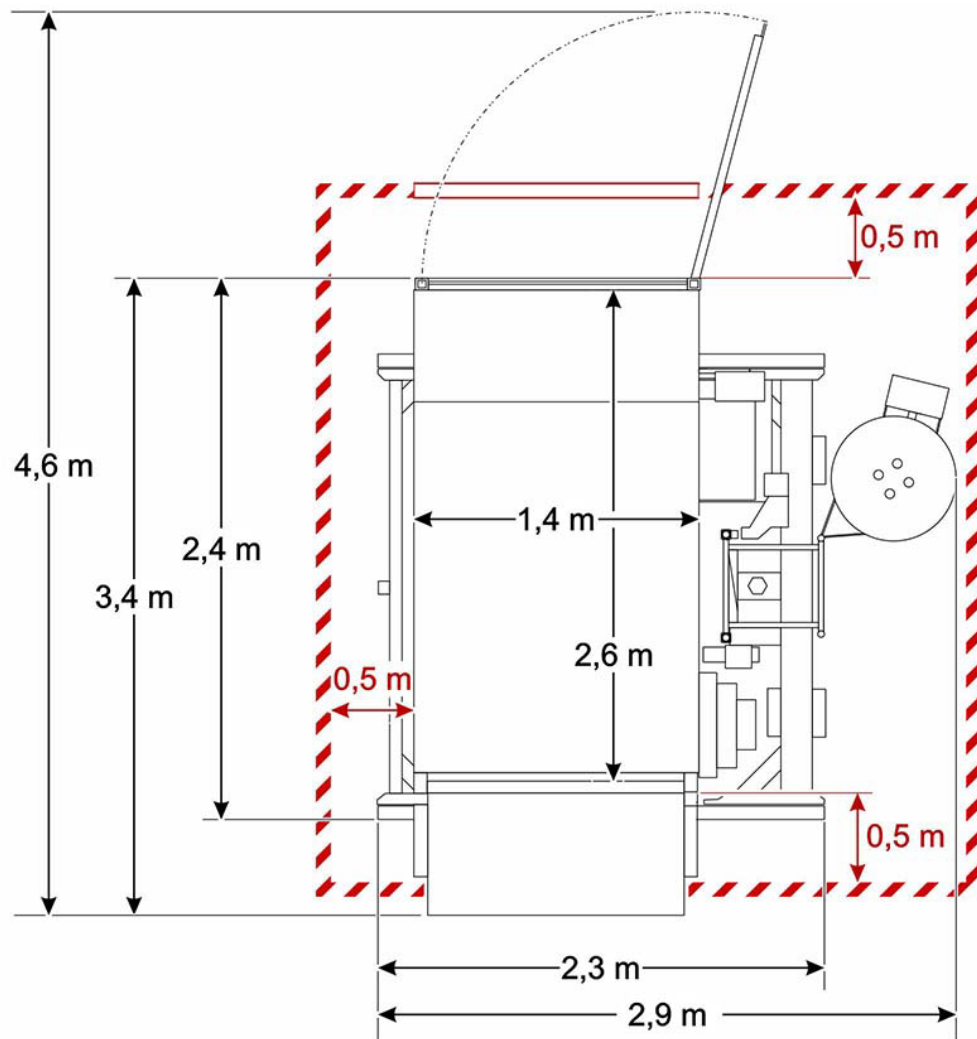
Abb. 7: Platzbedarf Bühne B
