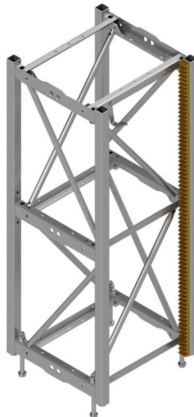
Abb. 2: S-VARIO MAST
