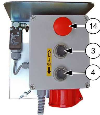
Abb. 56: Elektromodul für Etagensicherungstür
