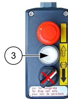
Abb. 78: Fangprobensteuerung
