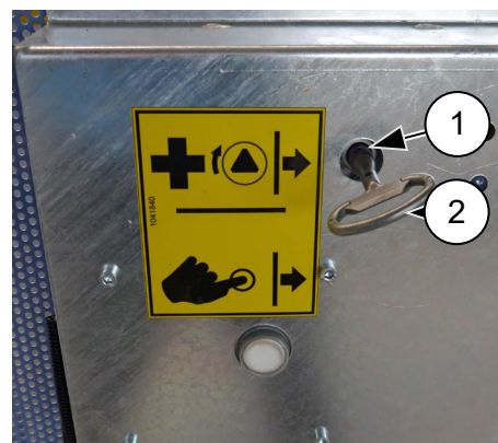
Abb. 24: Schiebetür Notentriegelung von außen
