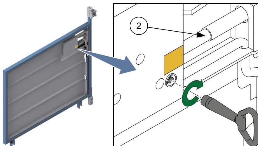
Abb. 34: Notentriegelung Rampe / Beladetür innen
