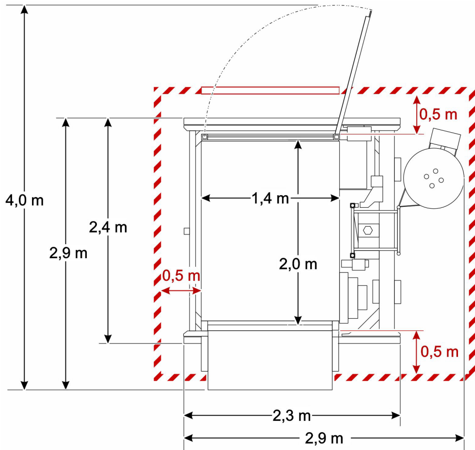
Abb. 5: Platzbedarf Bühne A
