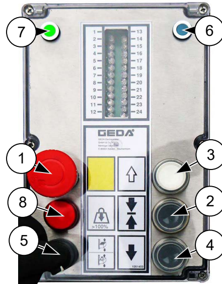
Abb. 80: Steuerung Bühne / Bedienung Transportbühne
