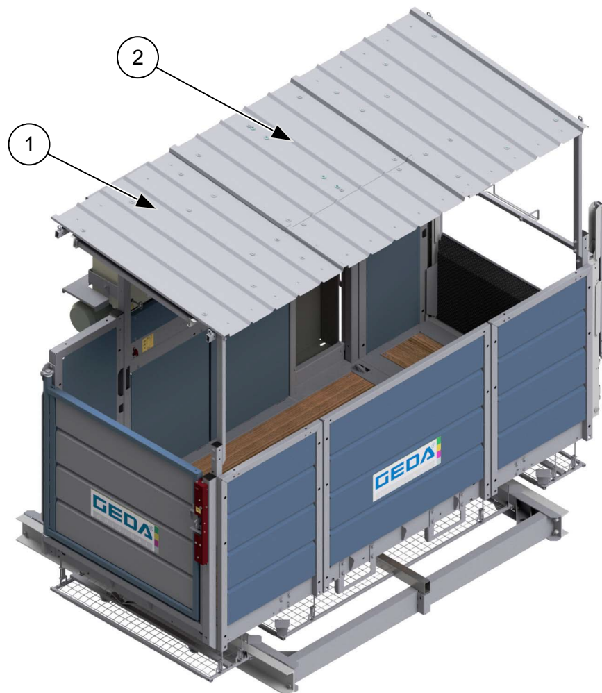
Abb. 63: Dach mit einer Montageöffnung
