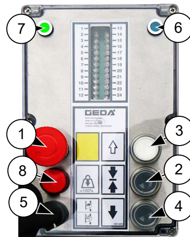
Abb. 57: Bühnensteuerung aktivieren
