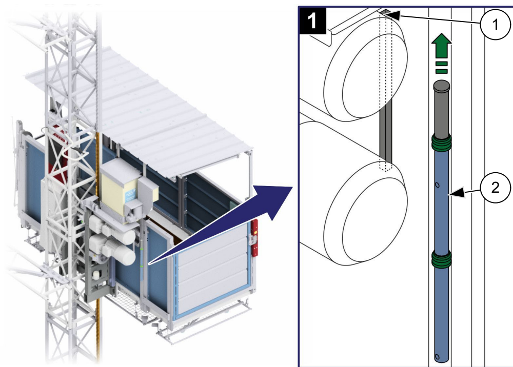
Abb. 81: Bremslüftstange mit Halterung
