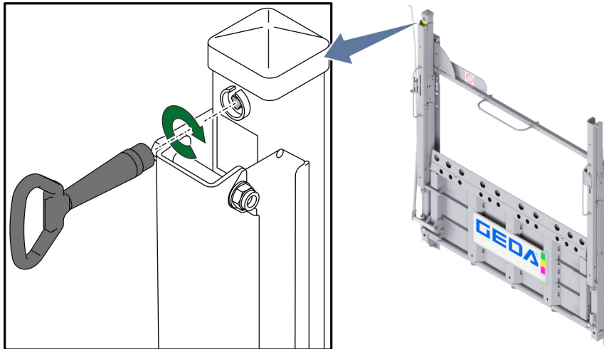
Abb. 38: Notentriegelung der Schranke mit elektromechanischer Verriegelung außen
