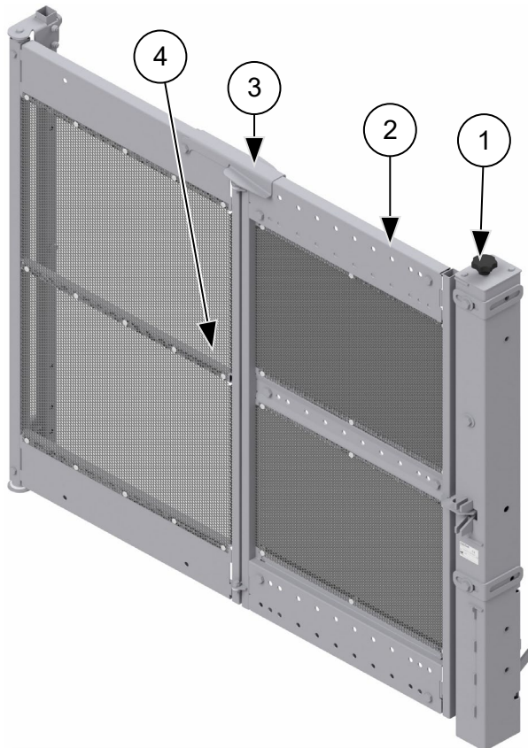
Abb. 50: Etagensicherungstür öffnen/schließen
