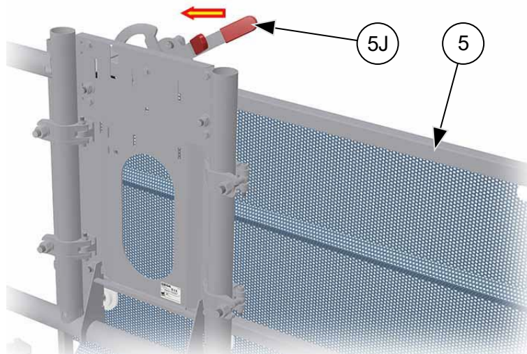
Abb. 49: Etagensicherungstür öffnen/schließen
