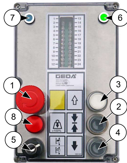
Abb. 76: Überlastanzeige
