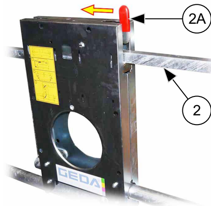
Abb. 47: Etagensicherungstür "Comfort" öffnen/schließen
