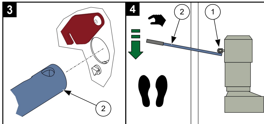
Abb. 83: Bremslüftung ziehen
