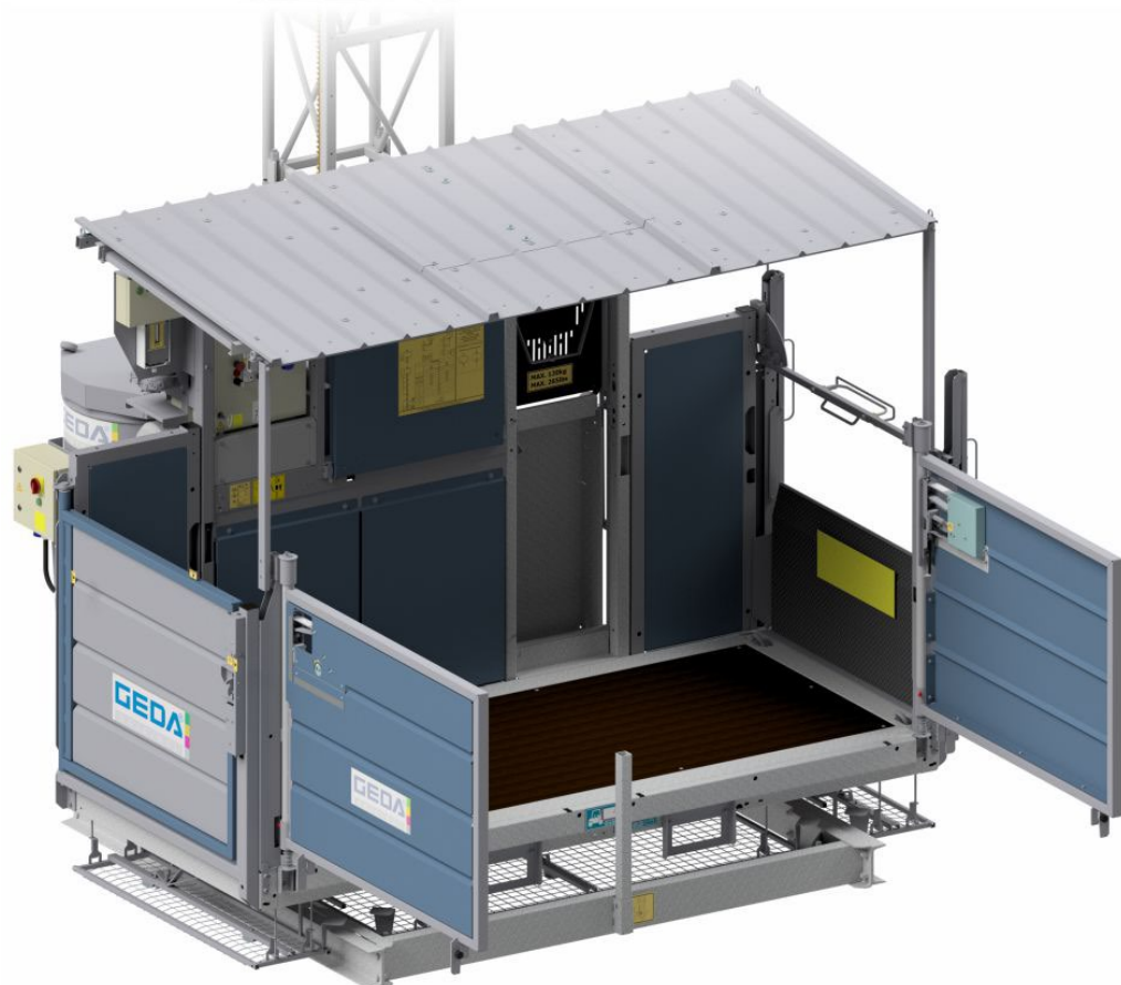
Abb. 31: Bühnenzugang Frontseite
