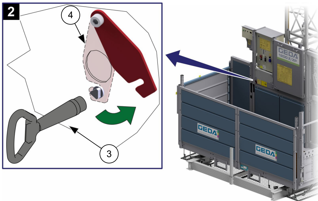
Abb. 82: Öffnung für Bremslüftstange
