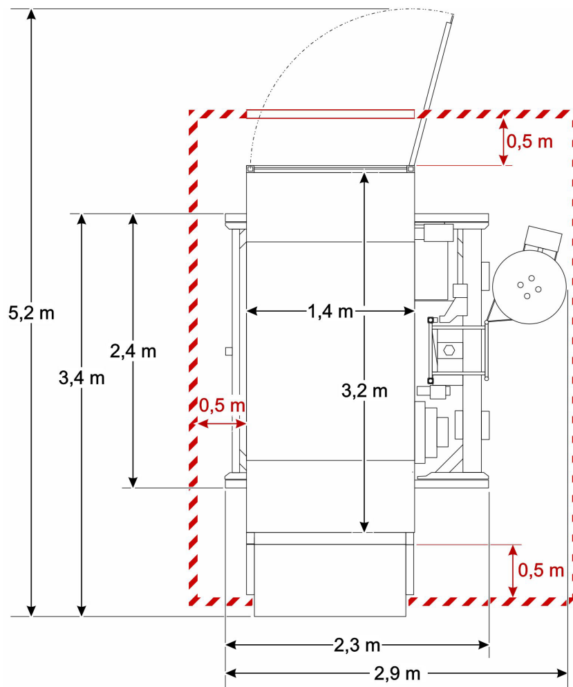
Abb. 9: Platzbedarf Bühne C
