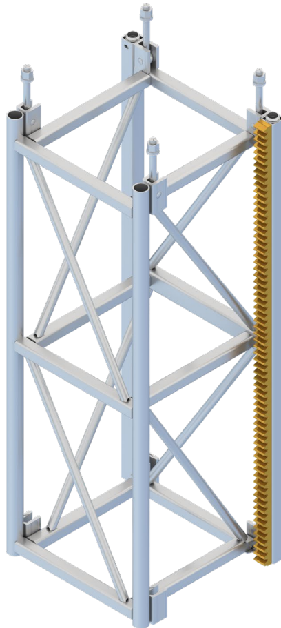
Abb. 1: VARIO MAST
