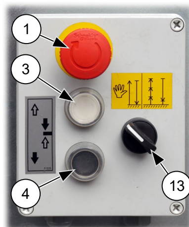
Abb. 53: Bodensteuerung für Umwehung (HAND)
