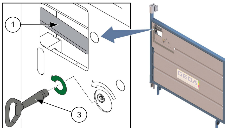
Abb. 33: Notentriegelung Rampe / Beladetür außen
