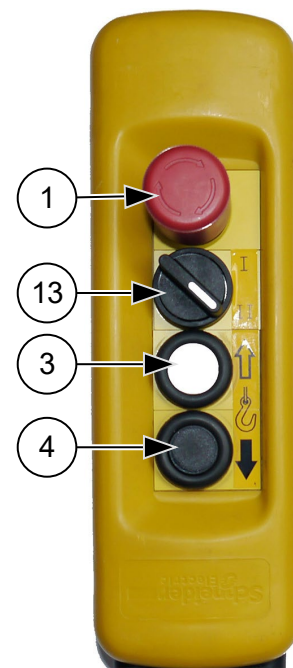
Abb. 54: Bodensteuerung/Handsteuerung (Stellung II)
