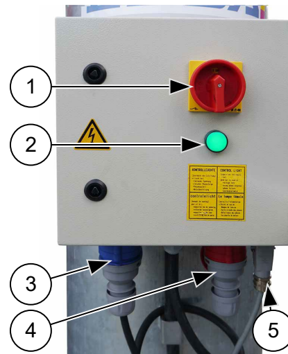
Abb. 14: Schaltkasten Bodenstation
