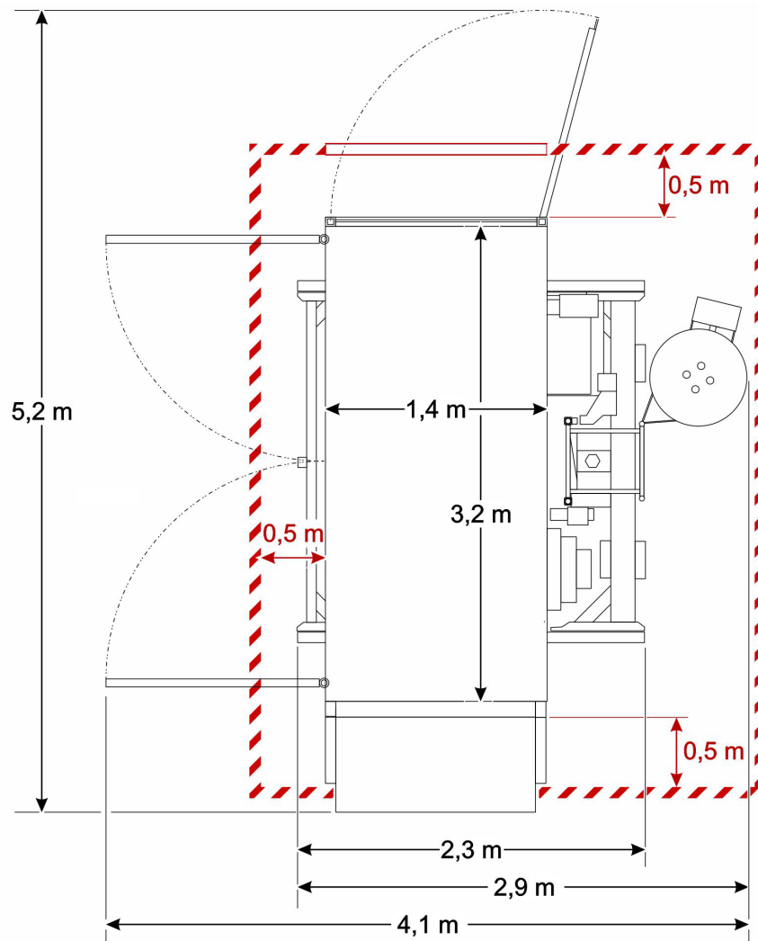
Abb. 13: Platzbedarf Bühne C mit Flügeltür
