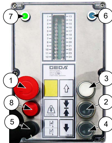
Abb. 59: Bühnensteuerung zur Montage
