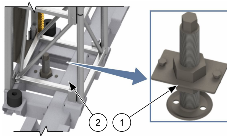
Abb. 73: Zentralspindel montieren
