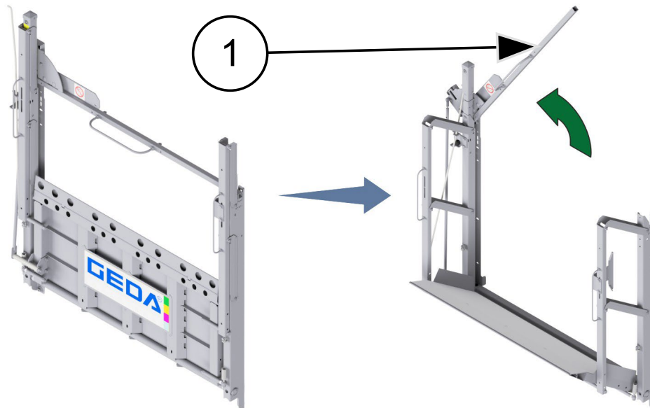
Abb. 37: Schranke mit elektromechanischer Verriegelung öffnen/schließen
