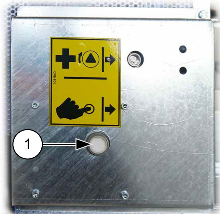
Abb. 20: Schiebetür Schloss entriegeln
