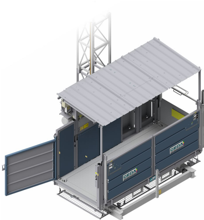
Abb. 27: Bühnenzugang Bodenstation
