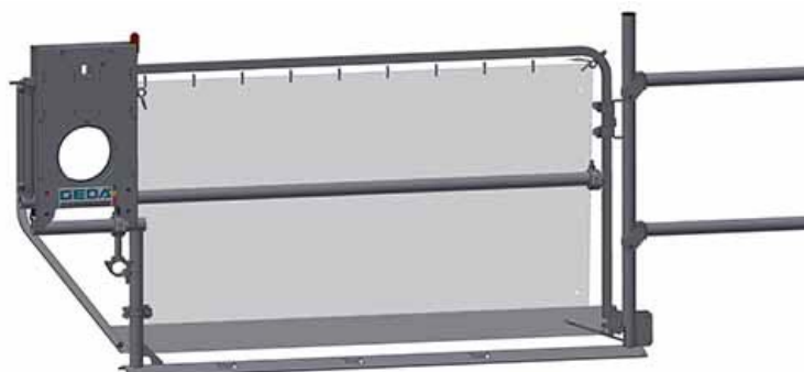
Abb. 42: Etagensicherungstür "Standard" geschlossen (Plane)
