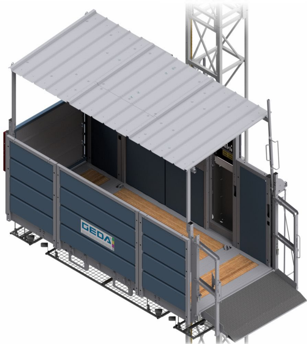
Abb. 35: Bühnenzugang Etage
