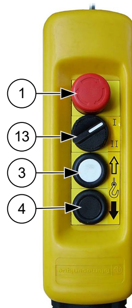
Abb. 52: Bodensteuerung/Handsteuerung (Stellung I)
