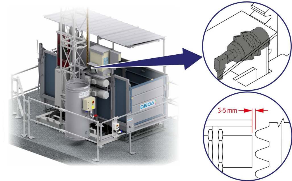
Abb. 66: Überfahr- und Kabelschutz
