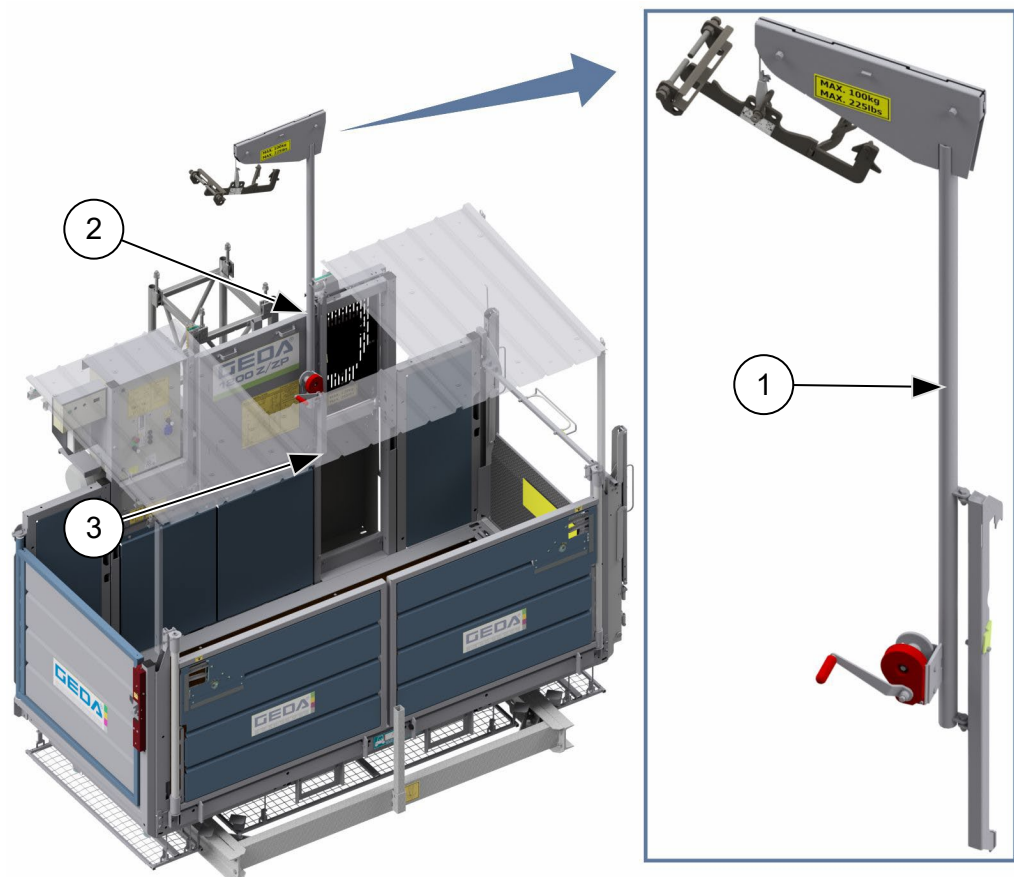
Abb. 72: Anheben, Positionieren von Mastteilen
