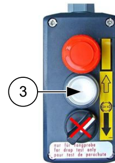
Abb. 75: Bedienung Fangprobensteuerung
