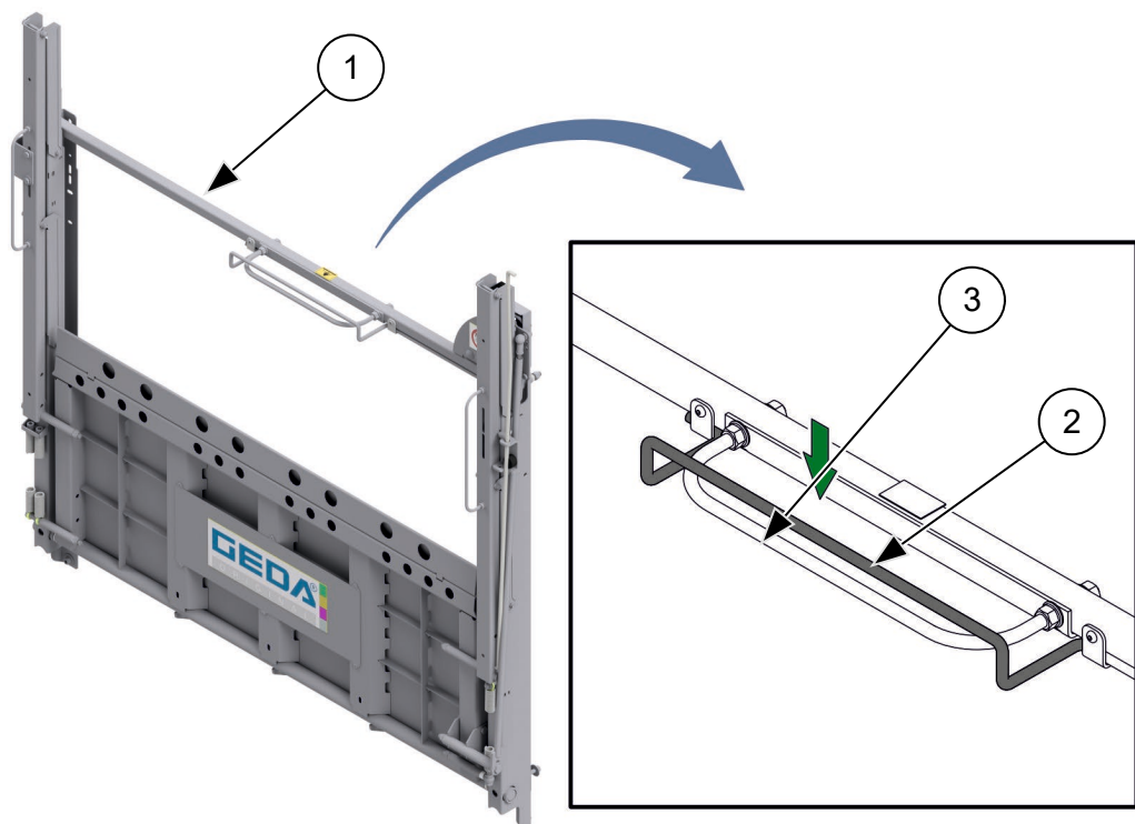
Abb. 36: Schranke mit mechanischer Verriegelung öffnen
