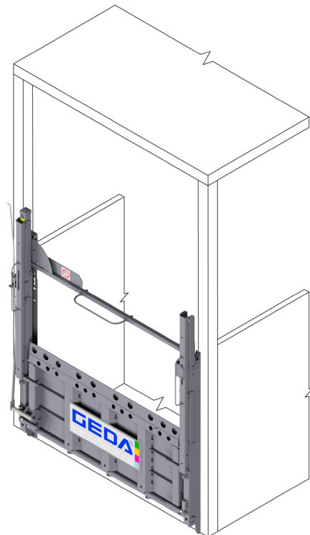
Abb. 27: Schranke mit elektromechanischer Verriegelung
