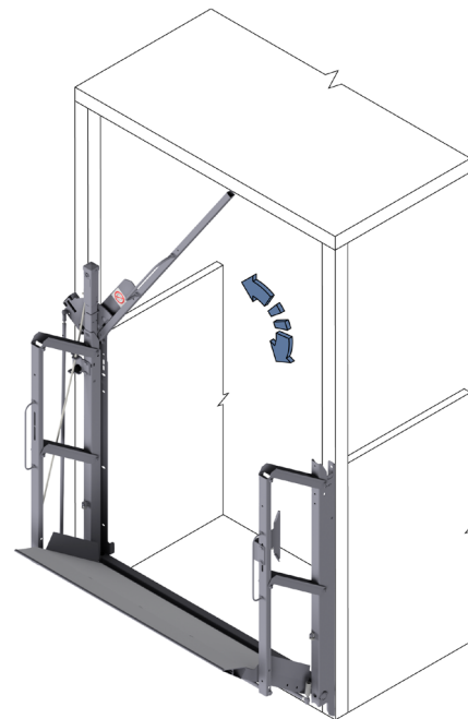
Abb. 28: Schranke mit elektromechanischer Verriegelung öffnen/schließen
