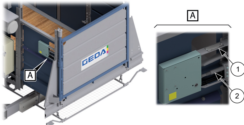
Abb. 19: Beladetür Verriegelung
