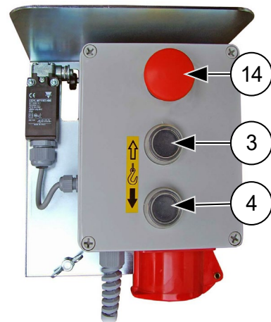
Abb. 44: Elektromodul für Etagensicherungstür
