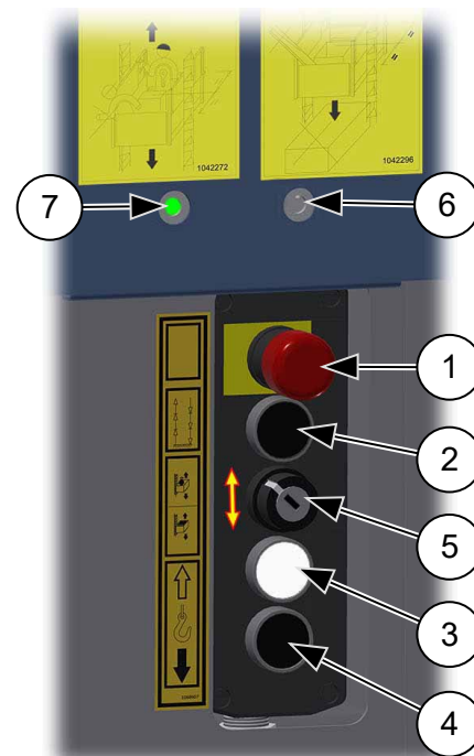
Abb. 47: Bühnensteuerung zur Montage
