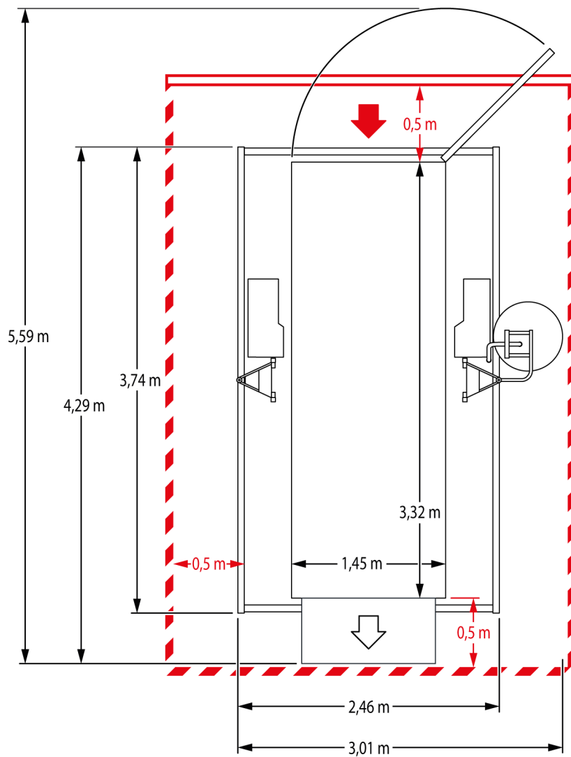
Abb. 5: Platzbedarf Bühne BS
