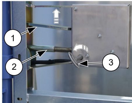
Abb. 20: Notentriegelung Rampe / Beladetür außen
