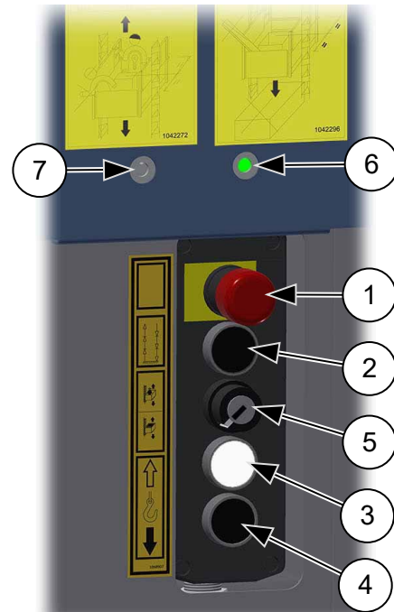
Abb. 39: Außensteuerung aktivieren
