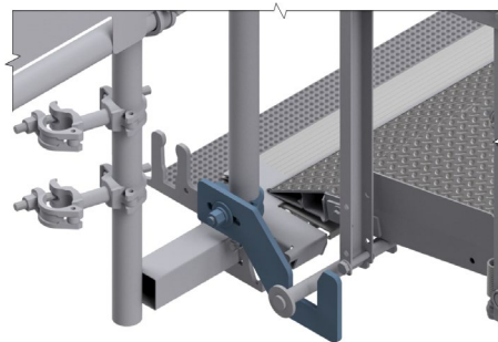
Abb. 38: Fanghaken für Etagensicherungstür
