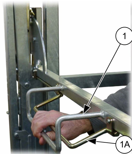
Abb. 25: Schranke mit mechanischer Verriegelung öffnen
