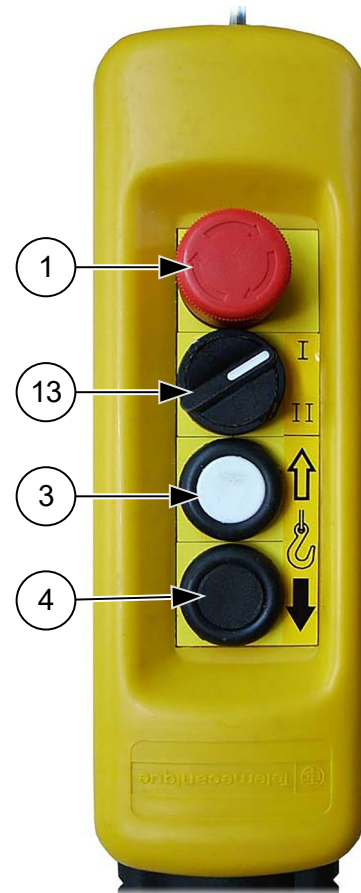
Abb. 40: Bodensteuerung/Handsteuerung (Stellung I)
