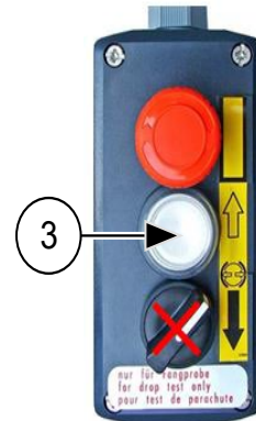
Abb. 63: Bedienung Fangprobensteuerung
