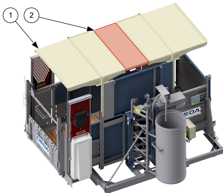
Abb. 51: Dach mit einer Montageöffnung
