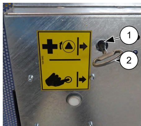
Abb. 16: Schiebetür Notentriegelung von außen
