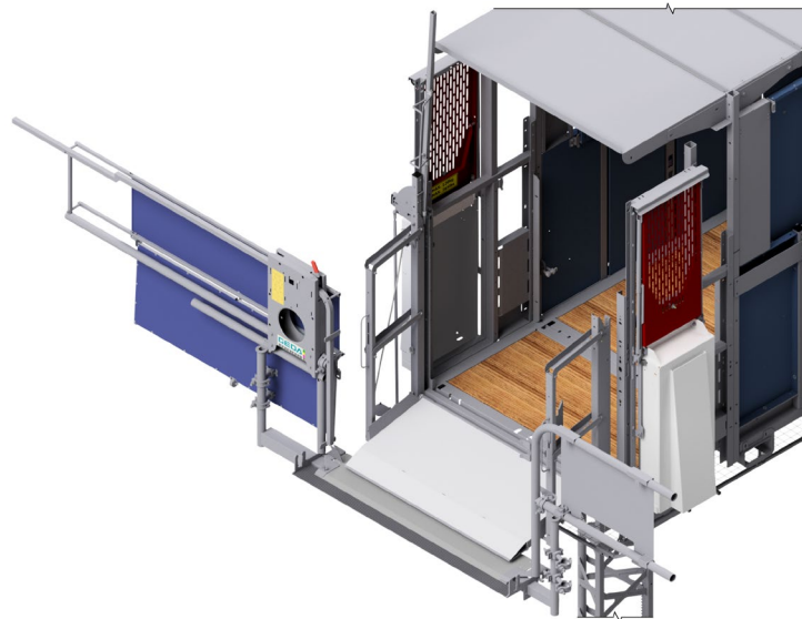
Abb. 23: Bühnenzugang Etage
