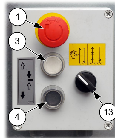
Abb. 41: Bodensteuerung für Umweh rung (HAND)
