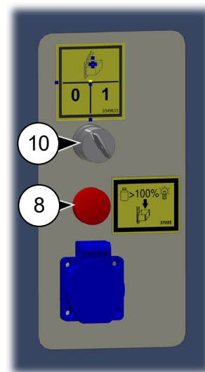
Abb. 7: Wahlschalter Betriebsart Betrieb
