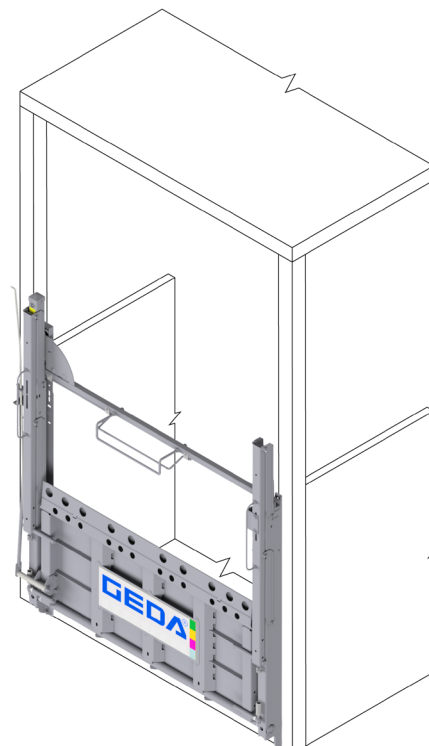
Abb. 24: Schranke mit mechanischer Verriegelung
