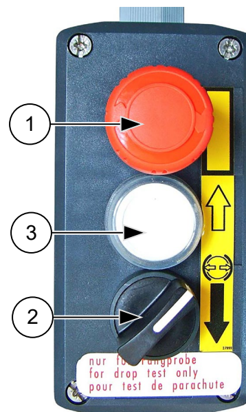
Abb. 48: Fangprobensteuerung
