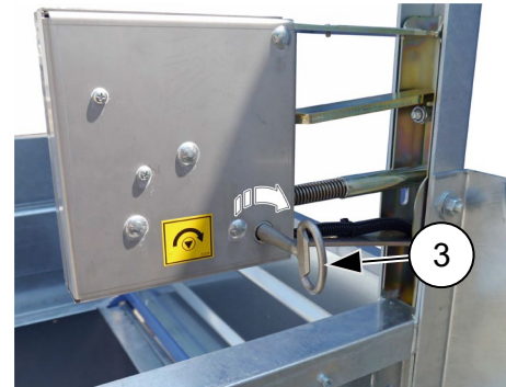
Abb. 21: Notentriegelung Rampe / Beladetür innen
