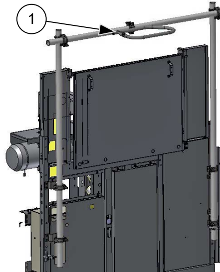
Abb. 57: Individueller Halter für Gerüstteile
