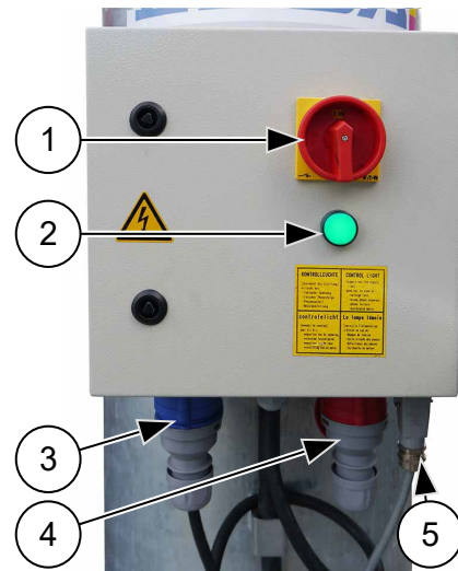
Abb. 6: Schaltkasten Bodenstation
