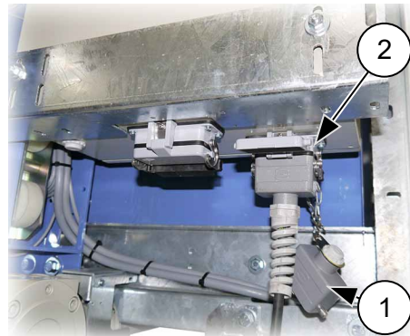
Abb. 65: Blindstecker Fangprobensteuerung
