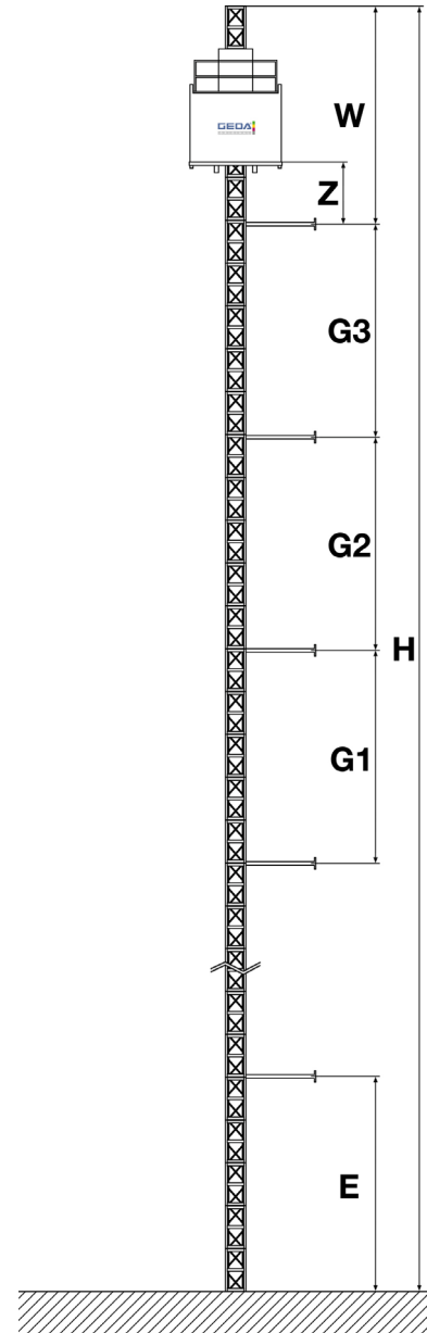
Abb. 3: Verankerung schematisch
