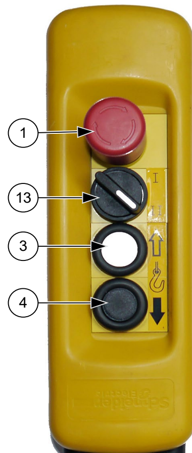
Abb. 42: Bodensteuerung/Handsteuerung (Stellung II)
