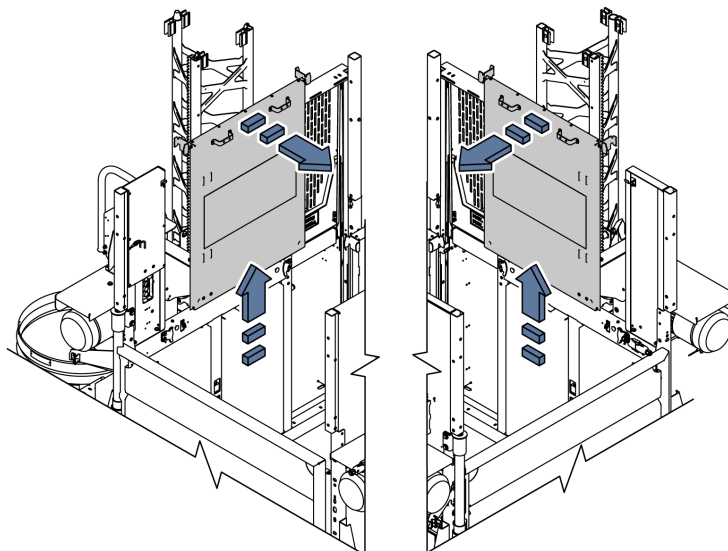
Abb. 70: Montageschutzblech demontieren
