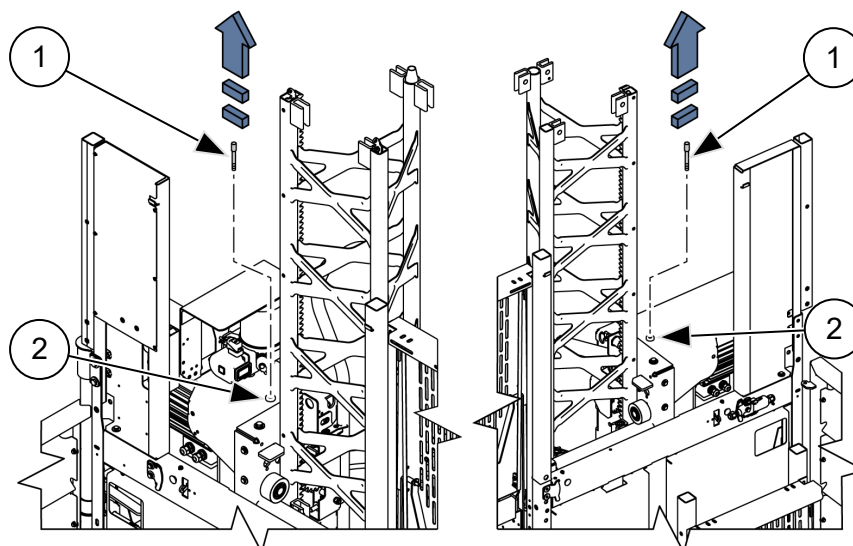
Abb. 71: Bremslüfthebel aus der Halterung nehmen
