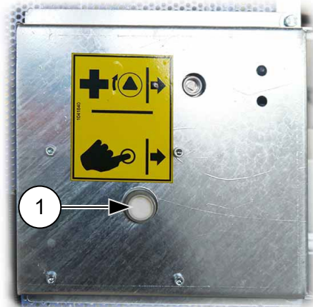
Abb. 12: Schiebetür Schloss entriegeln
