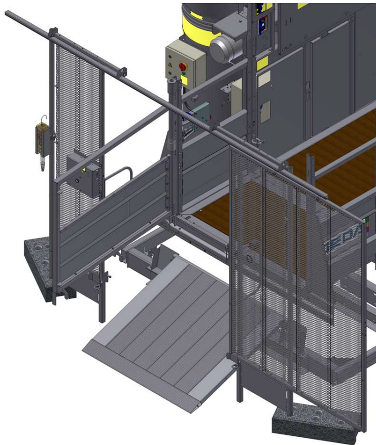
Abb. 15: Schiebetür für Bodenumwehrung geöffnet
