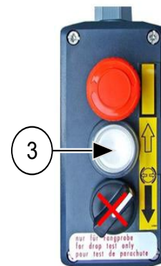
Abb. 66: Fangprobensteuerung
