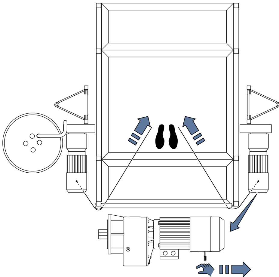
Abb. 74: NOT-Ablass ohne Umlenkeblech auslösen!
