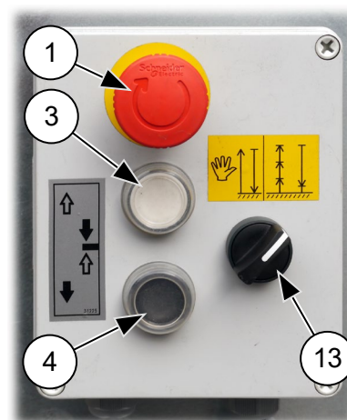
Abb. 43: Bodensteuerung für Umweh rung (AUTOMATIK)
