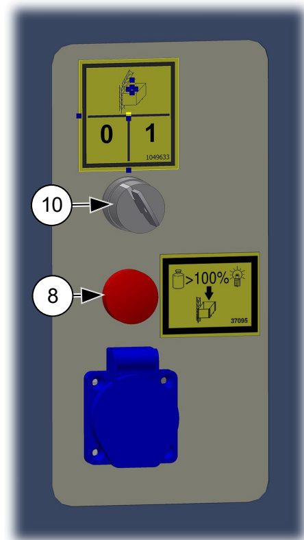
Abb. 64: Überlastanzeige
