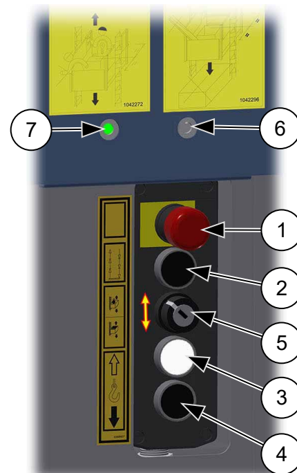
Abb. 68: Steuerung Bühne / Bedienung Transportbühne
