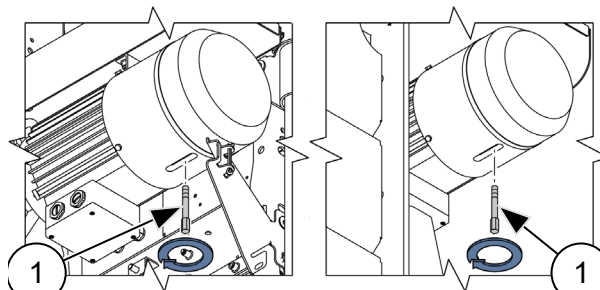
Abb. 72: Bremslüfthebel in die Motorbremse einschrauben
