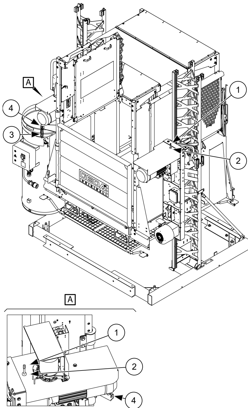
Abb. 69: Seil für Bremse lüften
