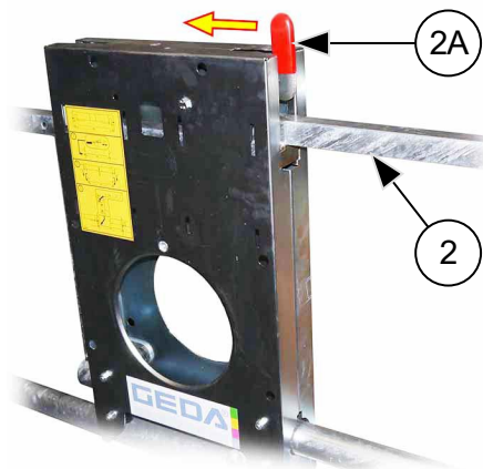
Abb. 37: Etagensicherungstür "Comfort" öffnen/schließen
