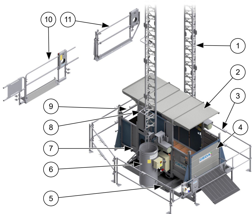
Abb. 8: Maschine Übersicht
