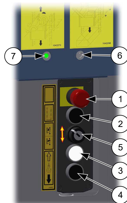
Abb. 45: Bühnensteuerung aktivieren
