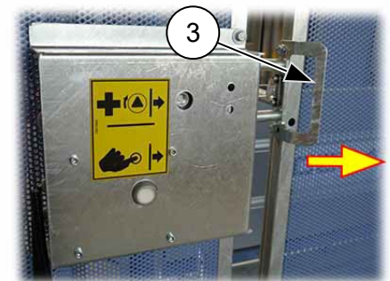
Abb. 14: Schiebetür schließen
