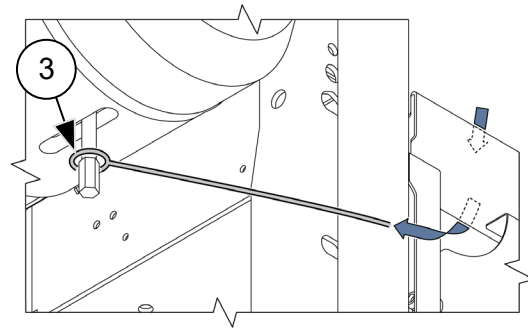
Abb. 73: Seilführung ohne Umlenkeblech
